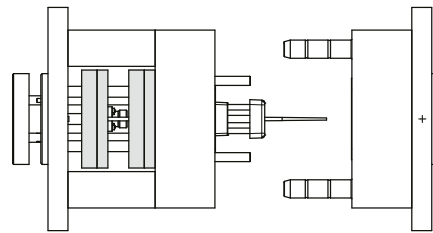
2.3 Curso 2: Separação dos dois conjuntos de placas de extração através do trinco interior redondo 313000. O conjunto de placas de extração 1 é mantido na posição. O conjunto de placas de extração 2 avança através do curso 2. Os extratores tubular e interior montados no conjunto de extração 2 desmoldam a peça de plástico. Recorrido 2: Separación de los dos paquetes de expulsión mediante el pestillo interior redondo 313000. El paquete de expulsión 1 se mantiene en su posición. El paquete de expulsión 2 avanza a través del recorrido 2. Los expulsos tubular e interior montados en paquete de expulsión 2 desmoldan la pieza de plástico.
