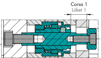
Tipo 1 (compatto)/Típus 1 (kompakt)
