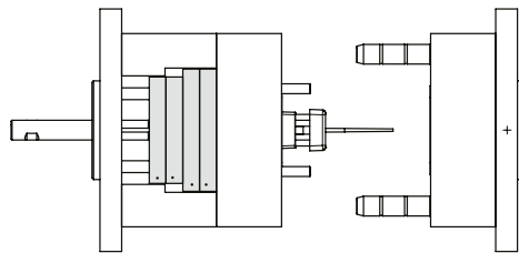
3.3 Corsa 2: il gruppo estrazione 2 resta fermo. Il gruppo estrazione 1 continua con la corsa 2. Il cannocchiale nel gruppo estrazione 1 espelle il particolare. 2. löket: Az 2. kidobócsomag megáll. A 1. kidobócsomag továbbhalad a 1. löketig. A 1. kidobócsomag hüvelye kilöki a műanyag alkatrészt.
