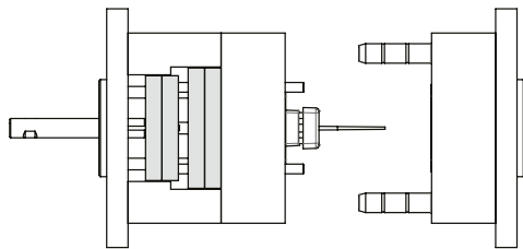
3.2 Corsa 1: i gruppi estrazione, posti a distanza costante, avanzano insieme di una corsa 1. L'asta inclinata libera il sottosquadro e solleva il particolare. Il cannocchiale nel gruppo estrazione 1 e l'estrattore nel gruppo estrazione 2 trattengono ancora il particolare. 1. löket: Mindkét kidobócsomag állandó távolságban mozdul előre 1 löketet. A ferde tolókar kiveszi a műanyag alkatrészt, amely felemelkedik. A hüvely a 1. kidobócsomagban és a kidobó a 2. kidobócsomagban még érintkezik az alkatrésszel.
