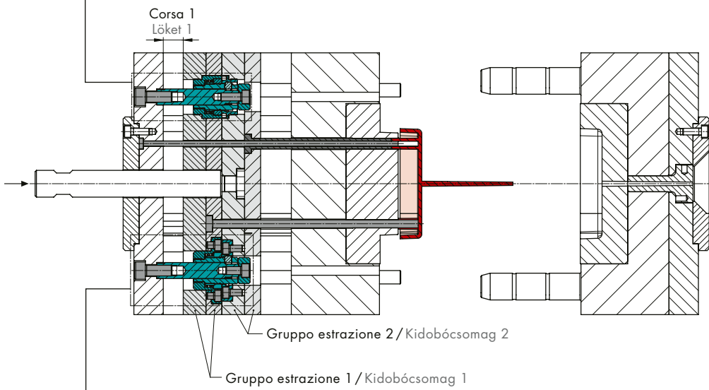
Tipo 1 (compatto)/Típus 1 (kompakt)
