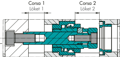
Tipo 1 (compatto)/Típus 1 (kompakt)
