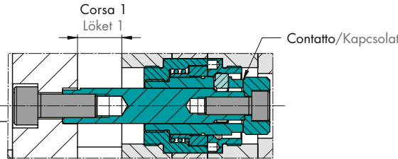
Tipo 1 (compatto)/Típus 1 (kompakt)
